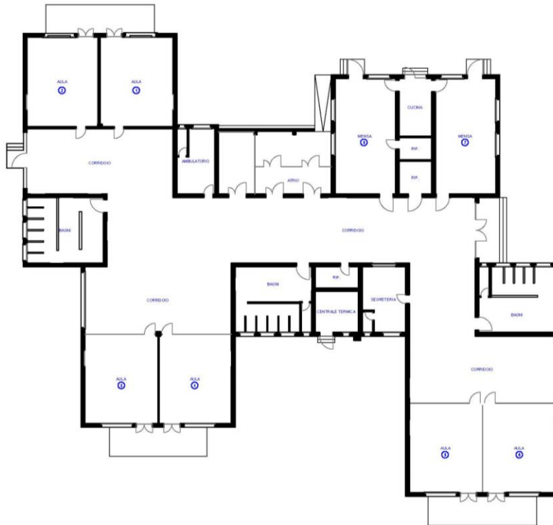
Planimetria 1: Locali piano terra
